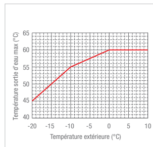
PUZ-WM60VAA / PUZ-WM85VAA
